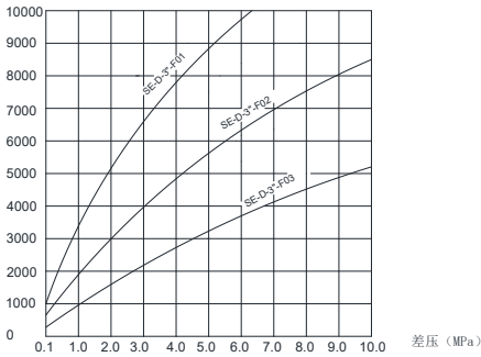
凝结水排量 (kg/h)
